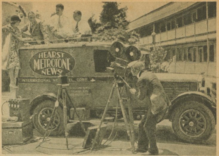
ЗВУКОВАЯ ПЕРЕДВИЖКА, УПОТРЕБЛЯЕМАЯ В АМЕРИКЕ ДЛЯ СЪЕМОК ЗВУКОВОЙ ХРОНИКИ И НАТУРНЫХ КАДРОВ
